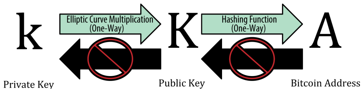
Figure 1. Clave privada, clave pública y dirección bitcoin
